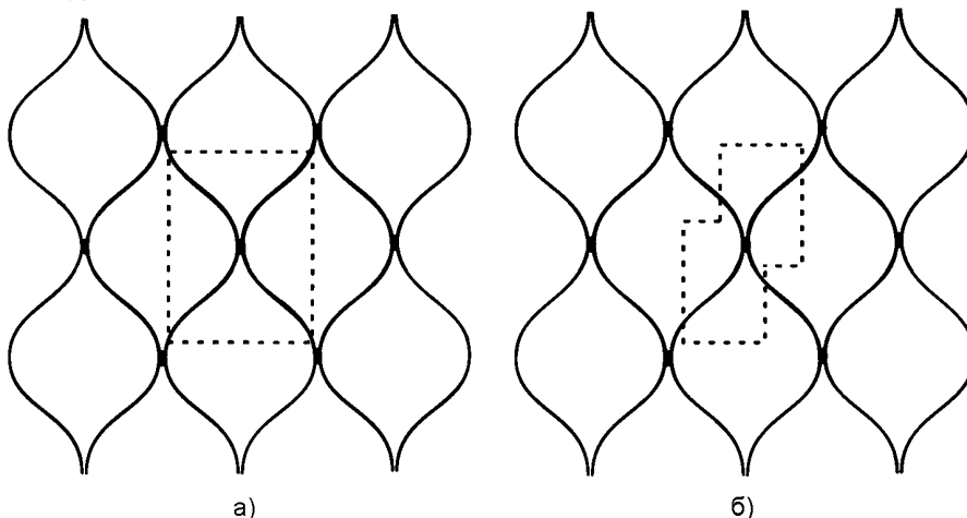
Рисунок 1 – Схема подготовки образцов при испытании на отрыв (а) и сдвиг (б)
